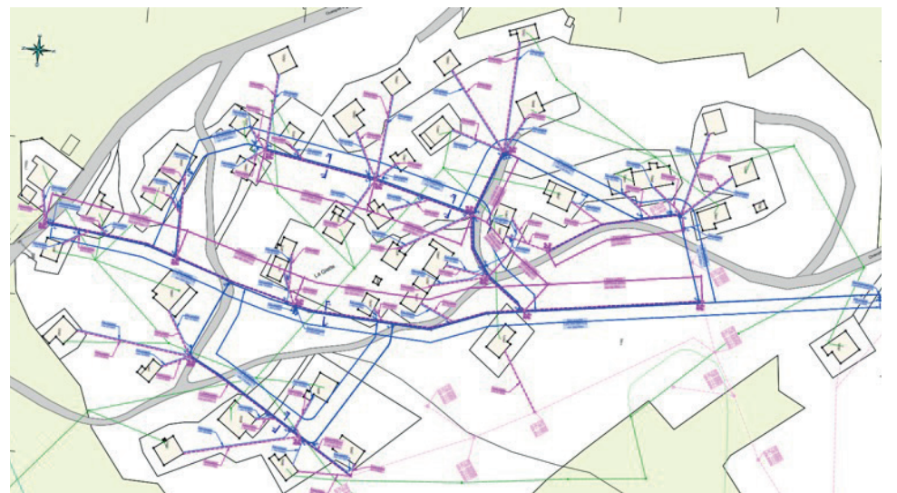
Plan des canalisations en phase d'avant-projet
